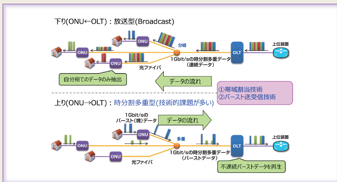
図5 PONの動作原理
