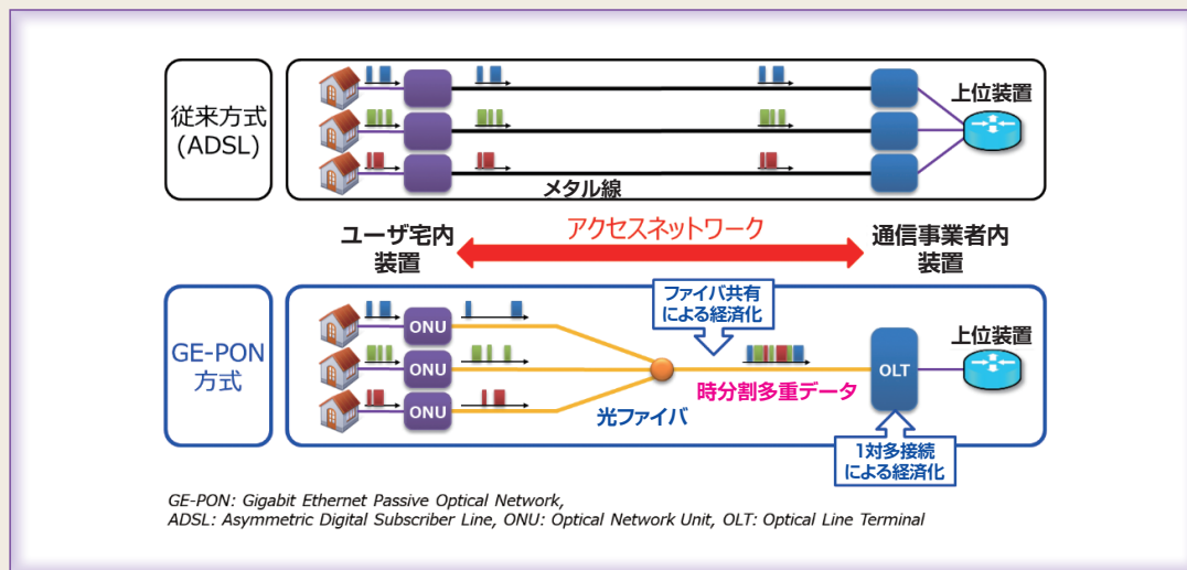
図2 DSLとPONシステムの比較図
