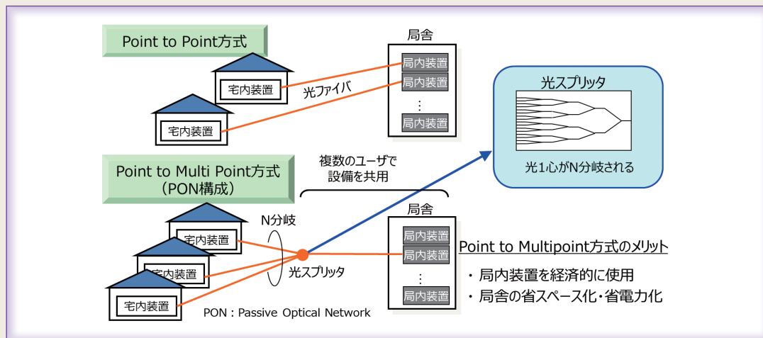
図3 光アクセスネットワークの形態
