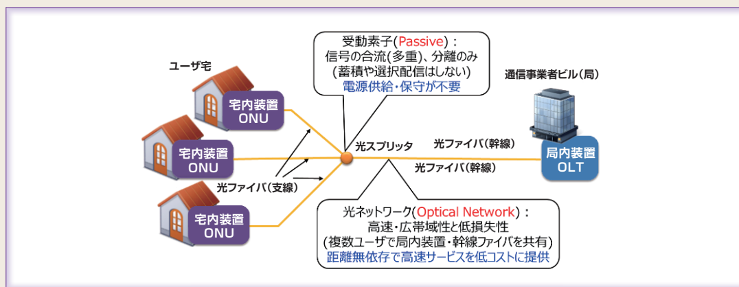
図4 PONシステムの基本構成及び主要な特徴
