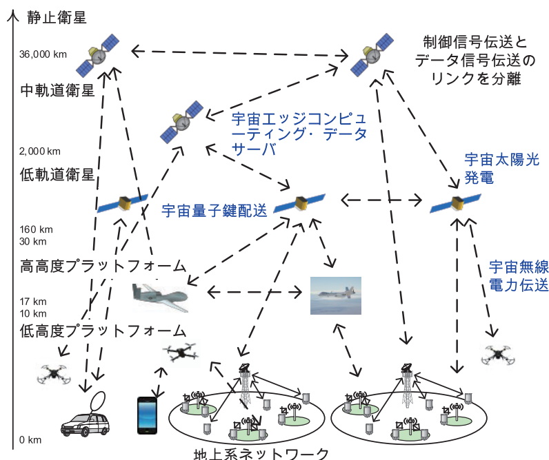
図3 6Gにおける宇宙統合ネットワーク
