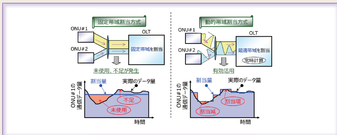
図6 帯域割当技術の概要
