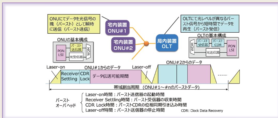
図8 OLT/ONU 基本構成とバーストデータフォーマット
