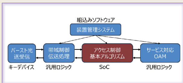
図10 OLT/ONUの機能構成図
