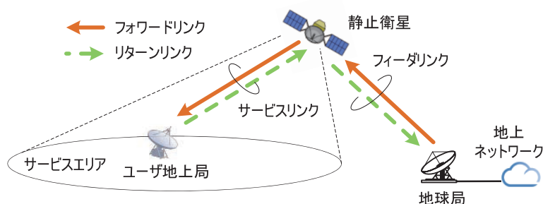
図1 静止衛星通信システム
