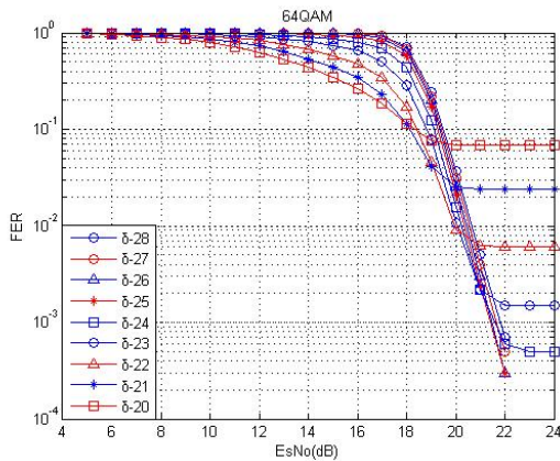
a. 64-QAM
