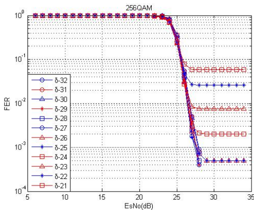
b. 256-QAM
