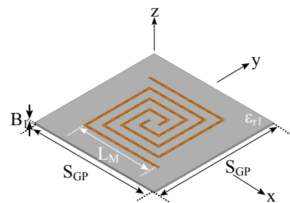
Fig. 1. Metaspiral antenna.
