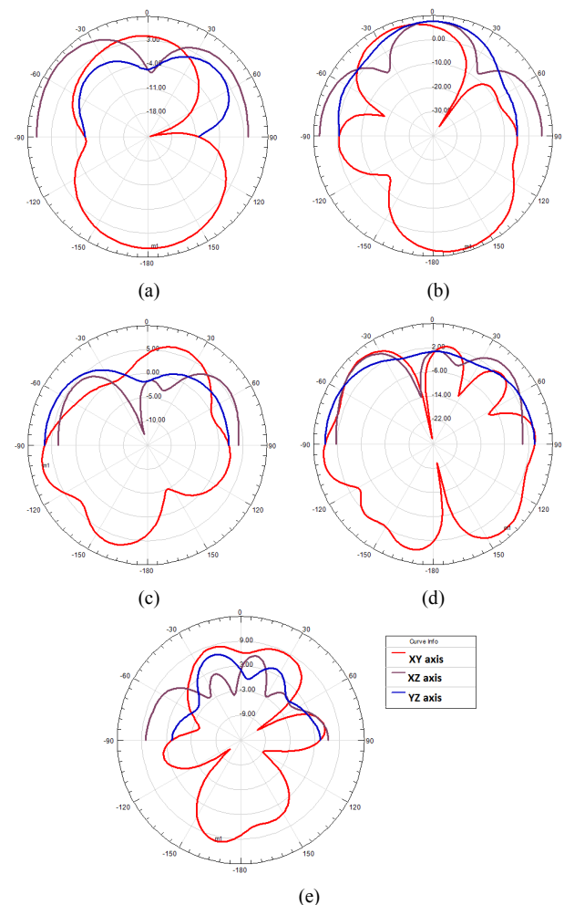
Fig. 4. Radiation Patterns at (a) 6.71GHz (b) 9.58GHz (c) 14.72GHz (d) 15.47GHz (e) 20.88GHz.
