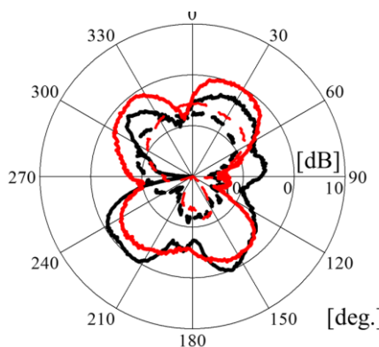
Fig. 6. Radiation pattern (yz-plane)
