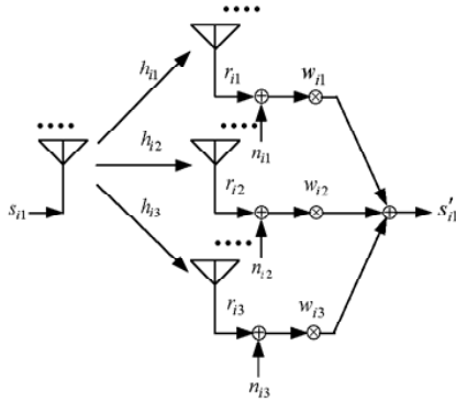
Fig. 2: 1x3 SIMO
