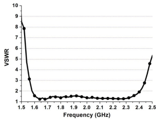
Fig. 2. VSWR.
