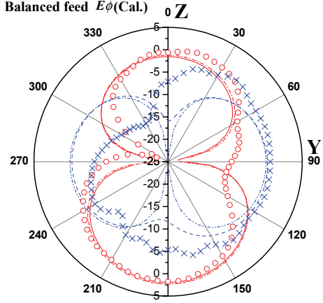
(a) 2.5GHz
