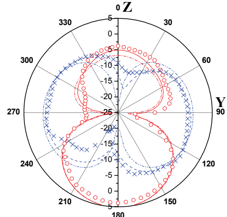
(b) 3.5GHz
