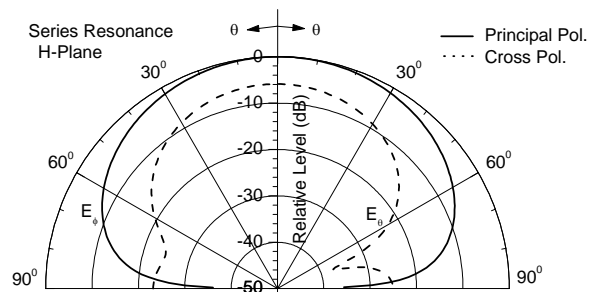
(b) H-Plane
