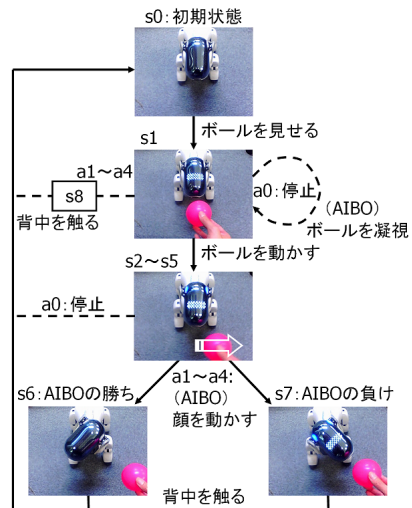
図 2: 学習における各状態とその遷移条件
