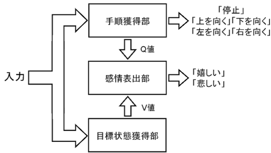
図 1: 学習システムの構成
