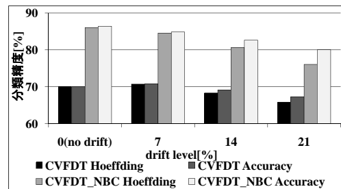
(a) 各組み合わせの分類精度 .
