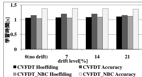
(b) 各組み合わせの学習時間 .
