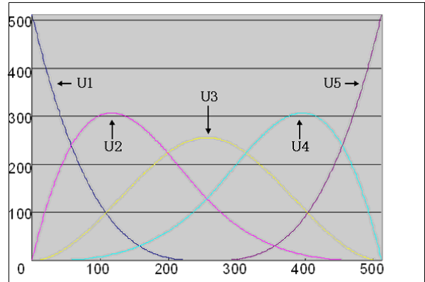
図7: u 方向の B-Spline 基底関数
