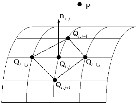
図5: 近点 Q_{ij} での接平面の法線ベクトル
