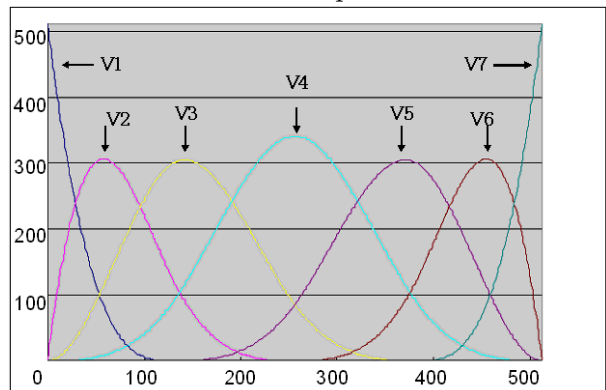
図7: u 方向の B-Spline 基底関数
