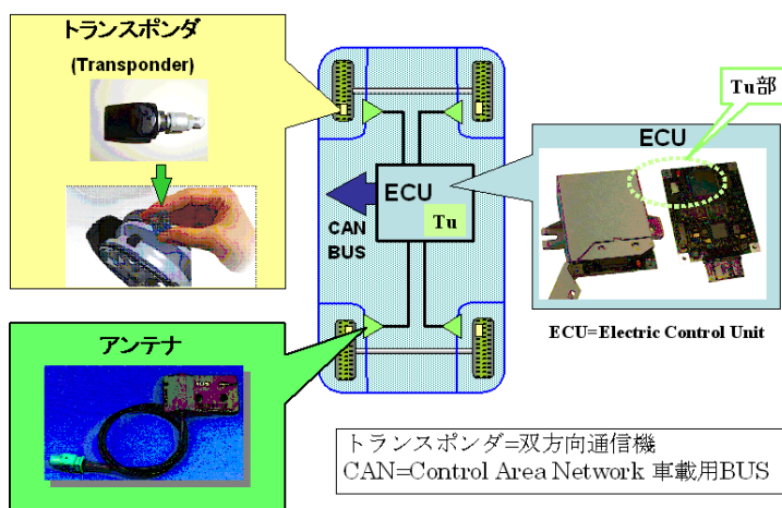
図 1: 電池レス TPMS システム
