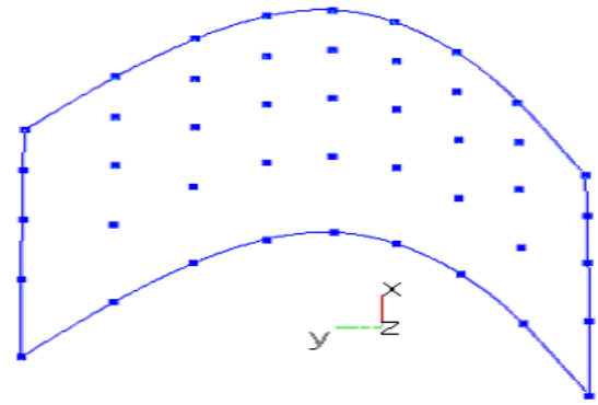
図 9: 初期入力点
