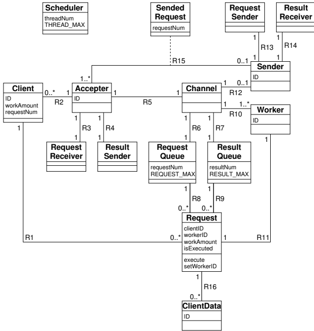
図 1: Worker Sender パターンのクラス図
