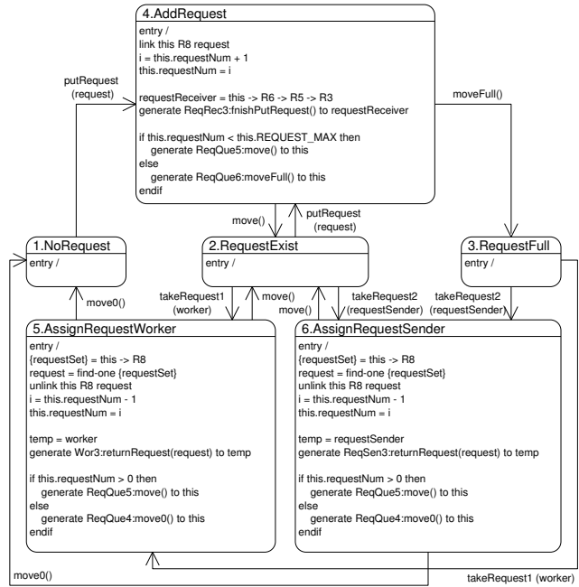
図 2: RequestQueue クラスの状態チャート図
