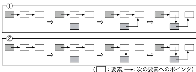
図 2: 単方向リストに要素を追加する例
