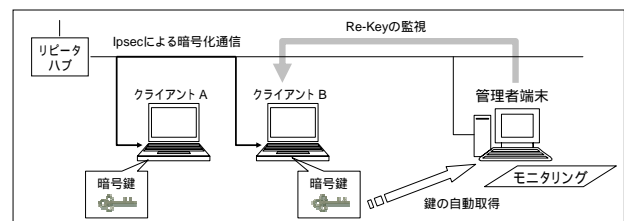
図 1. モニタリングシステムの構成
