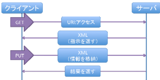
図 2. mobile-REST の制御シーケンス
