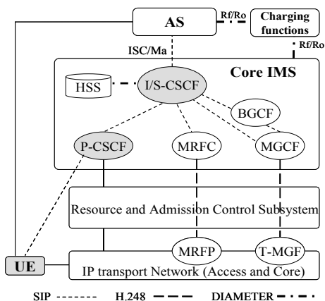
図 1. TISPAN-NGN の構成図
