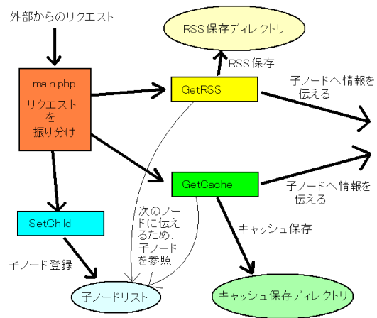
図 2: 各モジュールやコンテンツ間の関係
