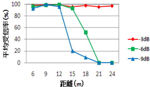
図5: 通信距離測定結果
