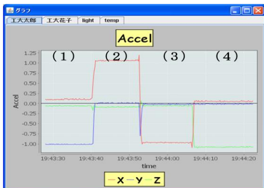
図7: 加速度グラフ
