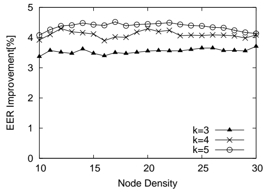
図 2: EER 改善率
