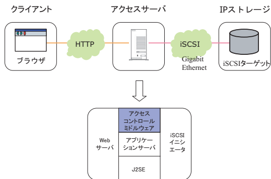
図 3: 実装環境とアクセスサーバの構成
