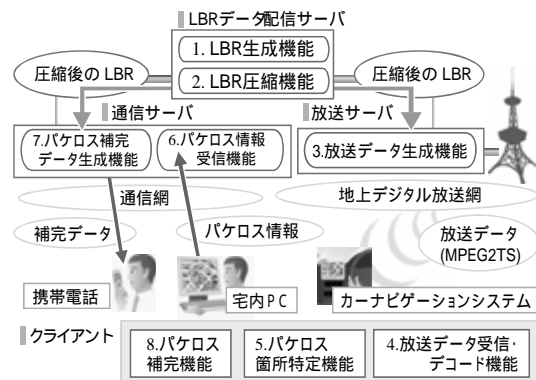
図1: 高度道路交通情報配信方式構成図
