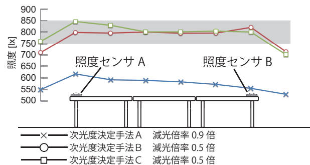
図6: グループ照明の中心を減光した際の各次光度決定手法による照度分布図
