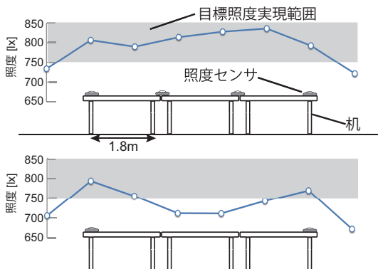
図 1: ANA/RC を用いた目標照度実現時の照度分布図
