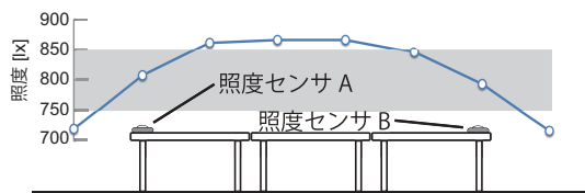
図4: 次光度決定手法Bによる収束時の照度分布図
