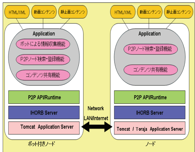
図3. ソフトウェア構成図
