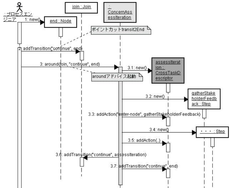
図7 アスペクト ConcernAssessment の織込み動作
