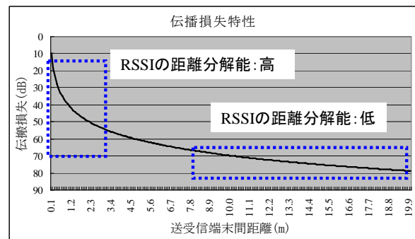
図 1 WLAN の伝搬損失特性
