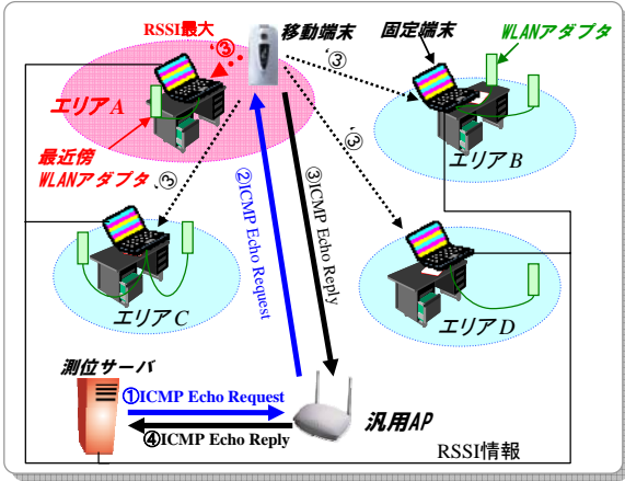
図2 送受信端末間距離の短縮方式
