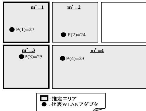
図5 複数エリアの推定例 (Pc=50)
