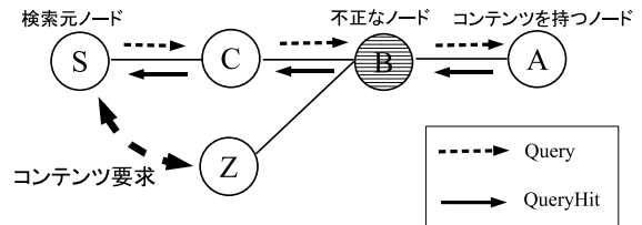
図 1: QueryHit の書き換え例
