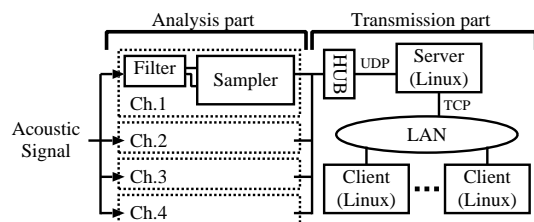
図 2: 音響構造配信システム
