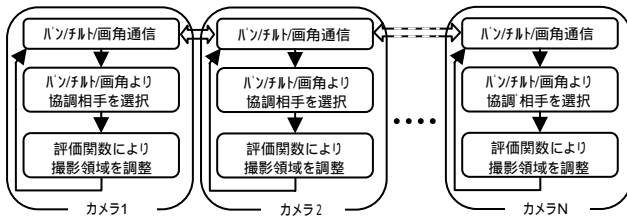
図2 処理フロー
