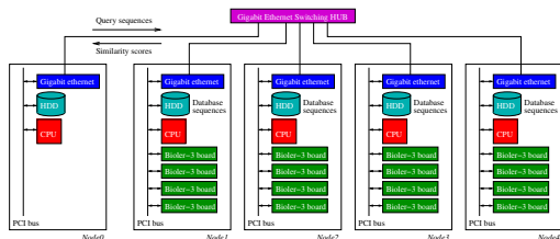
図 2: Bioler-3 を用いた PC クラスタシステム
