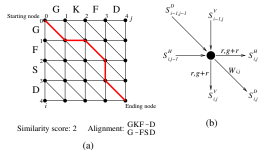
図1: DP ネットワークとノードにおける得点の流れ
