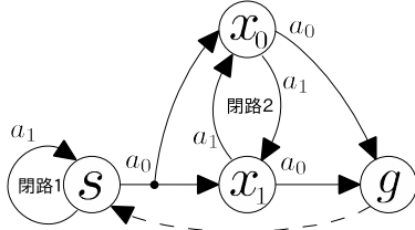
図 1: 閉路を含む単純な環境
