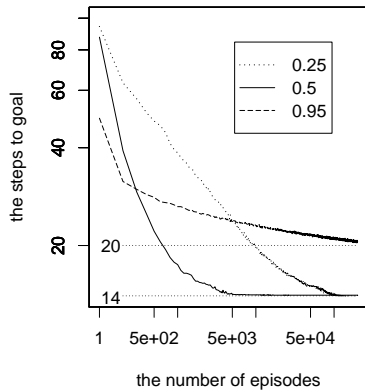
図 4: Dyna 迷路タスクにおける学習曲線
