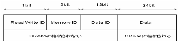
図 2 ID の構成
