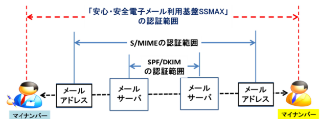
図2 SSMAXにおけるメール送信者の特定・追跡
