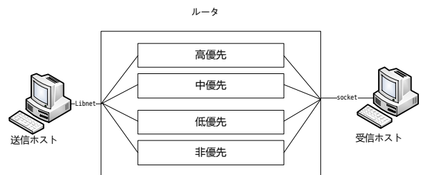
図2 システム構築
