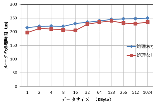
図 6 Flow Label を用いた優先度制御を実現したのルータ処理時間
