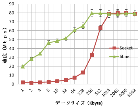
図 4 Libnet と Socket の通信速度
