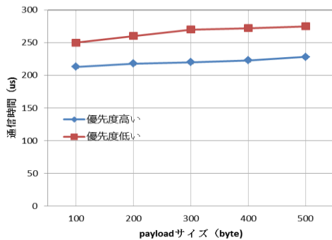
図 5 優先度の違うパケットの通信時間
