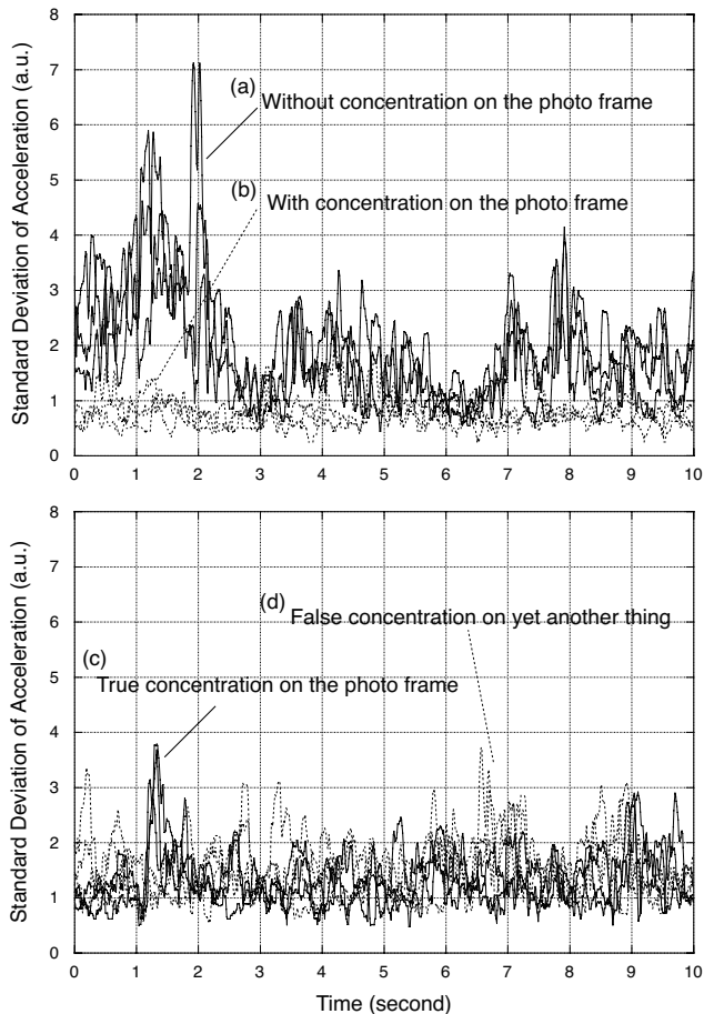
図2 16点加速度標準偏差値による運動の評価
