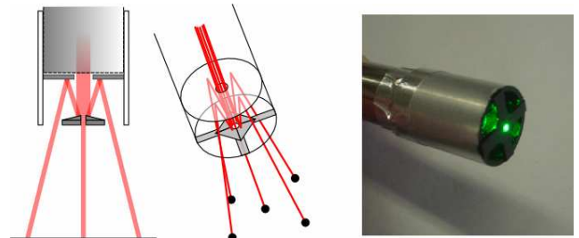
図2 レーザ光分岐アダプタ
