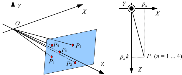
図3 レーザポインタ座標上の輝点
