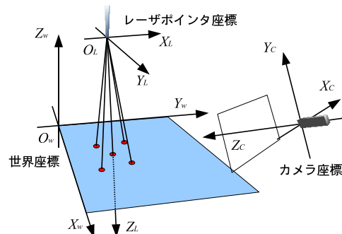
図1 世界座標、カメラ座標、レーザーポインタ座標
