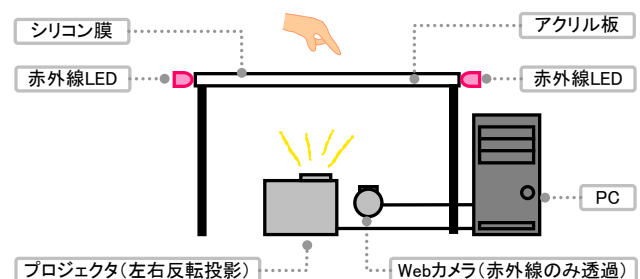
図 3-1 FTIR テーブルの構成
