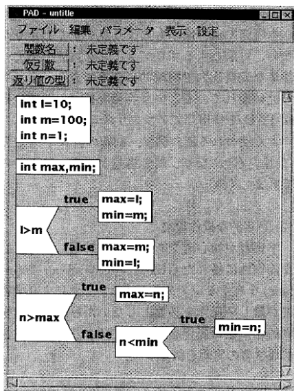
図 2 石田らの研究ツールの動作画面
