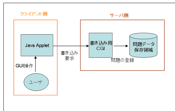
図6 システムの構成図
