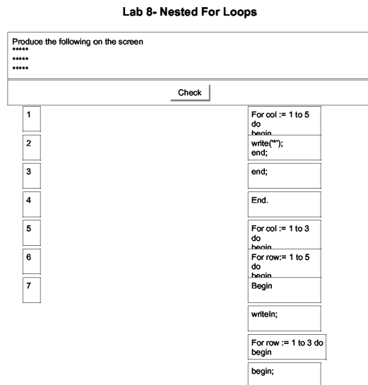
図 3 Parson's Programming Puzzles の動作画面:画面右に表示されているブロックを取捨選択しドラッグ&ドロップで画面左の数字欄にコードを並べ変えていく
