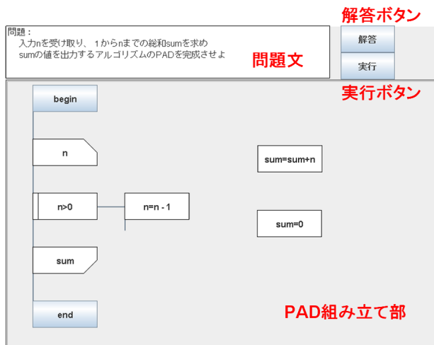
図4 提案システムの動作画面
