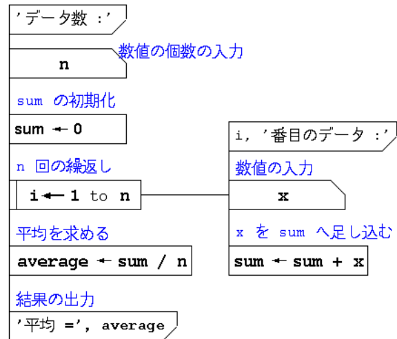
図 1 PAD 表示例：n 個の入力の平均値を求めるアルゴリズムの PAD を表している
