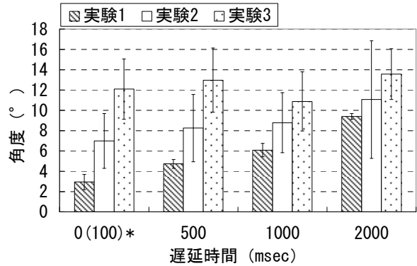
図 2: 遅延時間ごとの角度差の平均 (Yaw 軸回り) * (実験 3 において遅延 0msec は 100msec である)
