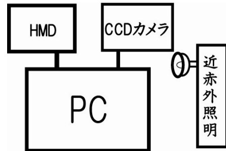
図 1. システムのブロック図
