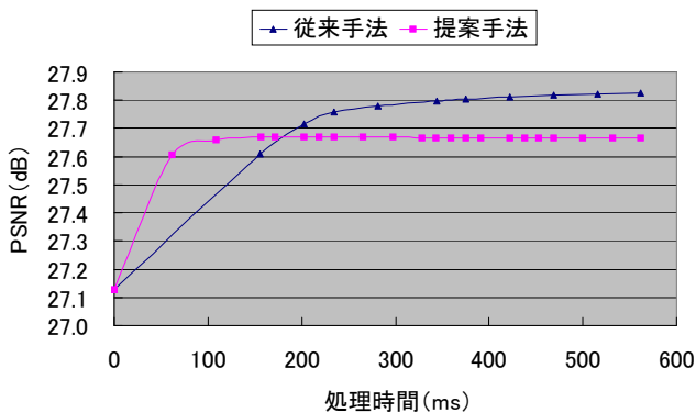
図 3 処理時間と PSNR の関係 (airplane)
