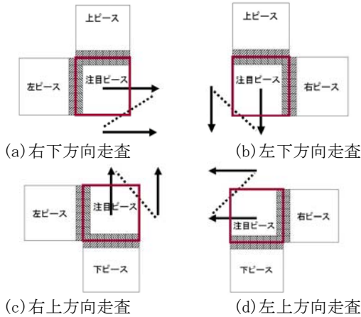
図3 マルチスキャンにおける注目ピースと隣接の参照ピース
