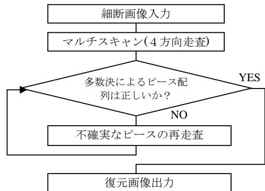
図 2 全体の流れ図
