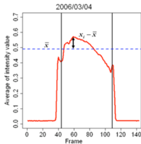
図4 日の出から日の入りまでの明度値の標準偏差導出
