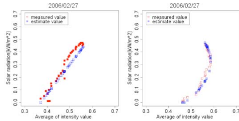
図5 ある一日における日射量と画像の明度値との関係
