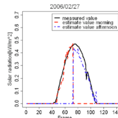
図7 計測された日射量と推定値との比較
