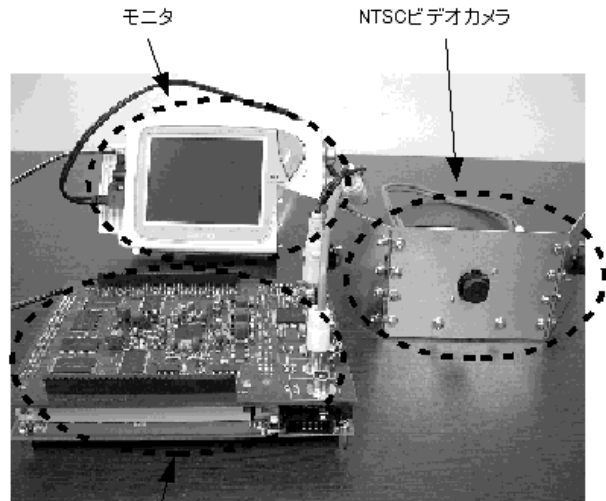
ビデオ信号入力出力ボード及びFPGA搭載ボード
