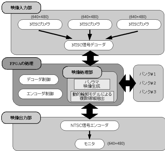
図 2: 全体の構成図
