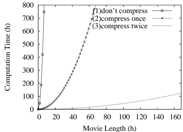
図 4: 長時間映像に適用したときに予測される計算時間
