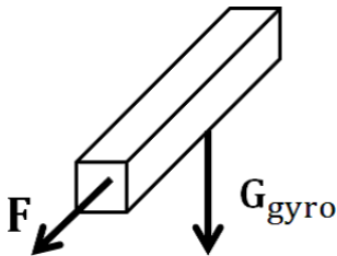
図 2: 正面方向のベクトルと重力方向のベクトル
