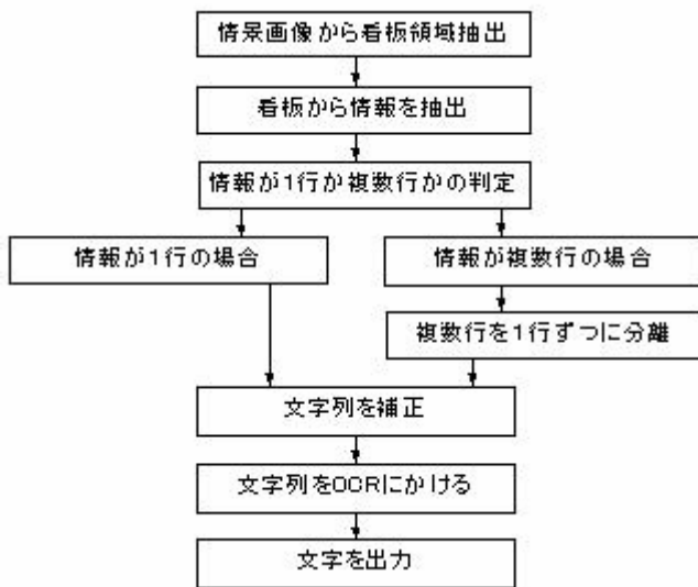
図1 看板認識システムの流れ
