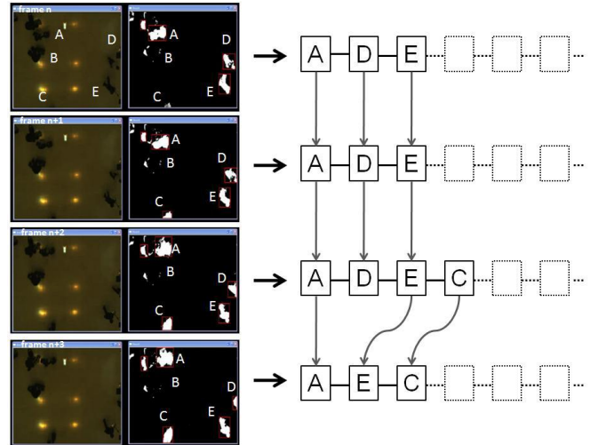
図1 ブロップトラッキングの例
