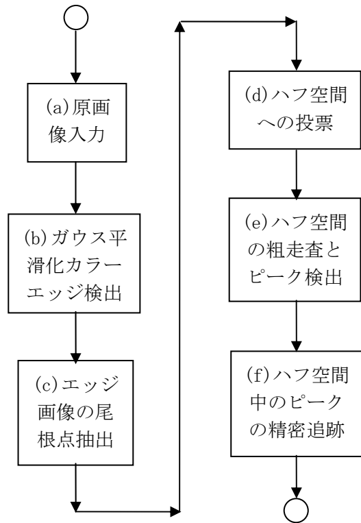
図1 ハフ変換に基づく人工物の直線検出の処理の流れ
