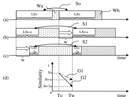
図1 アクティブセグメンテーションの原理
