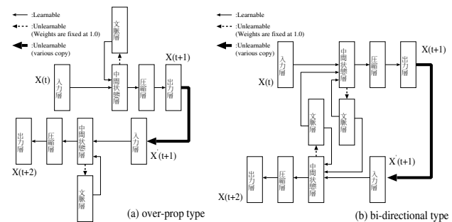
図 2: 2 段階予測モジュール
