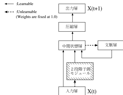
図 1: 提案する系列予測モデルの概要図
